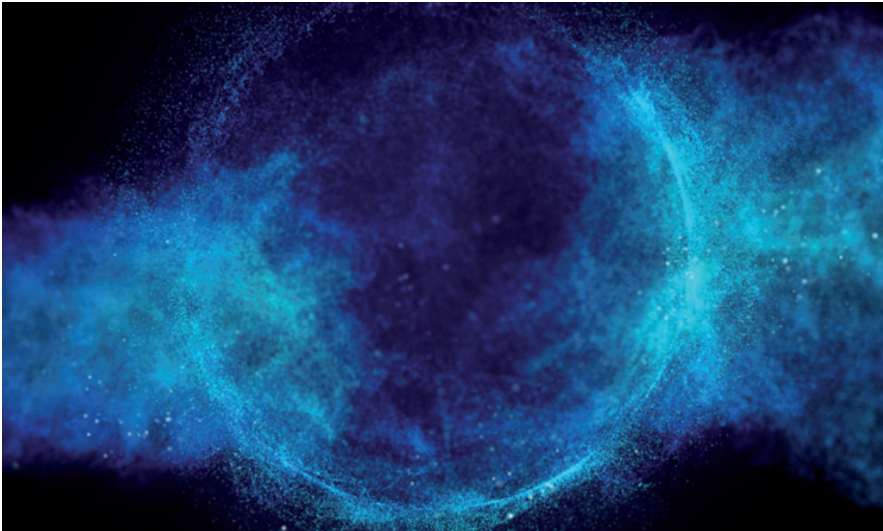
Καλλιτεχνική απεικόνιση του πεδίου Higgs (πηγή: CERN)
