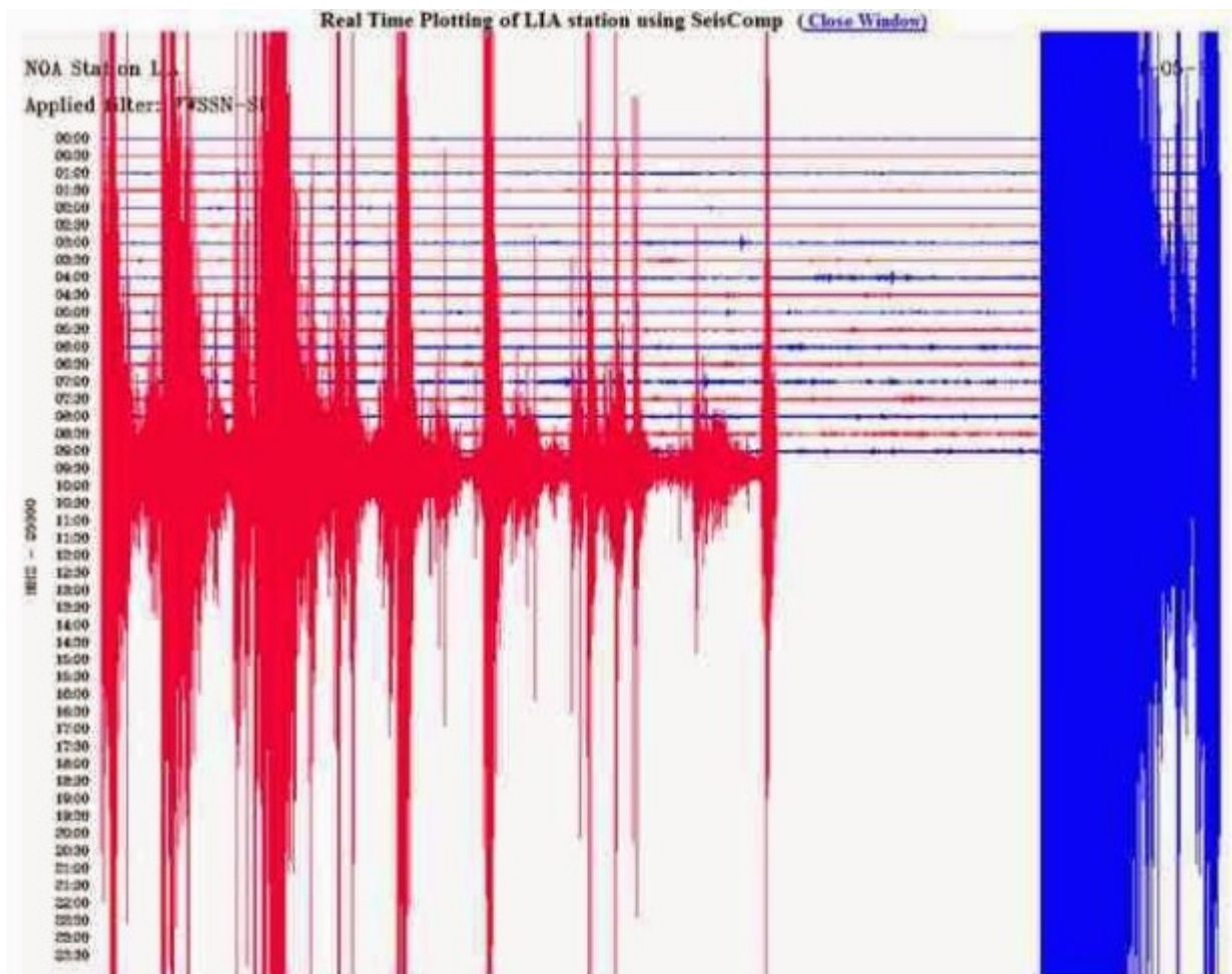
Δείτε πώς κατέγραψε τη δόνηση ο σειсмоγράφος του Γεωδυναμικού Ινστιτούτου του Εθνικού Αστεροσκοπείου Αθηνών που είναι εγκατεστημένος στη Λήμνο.
