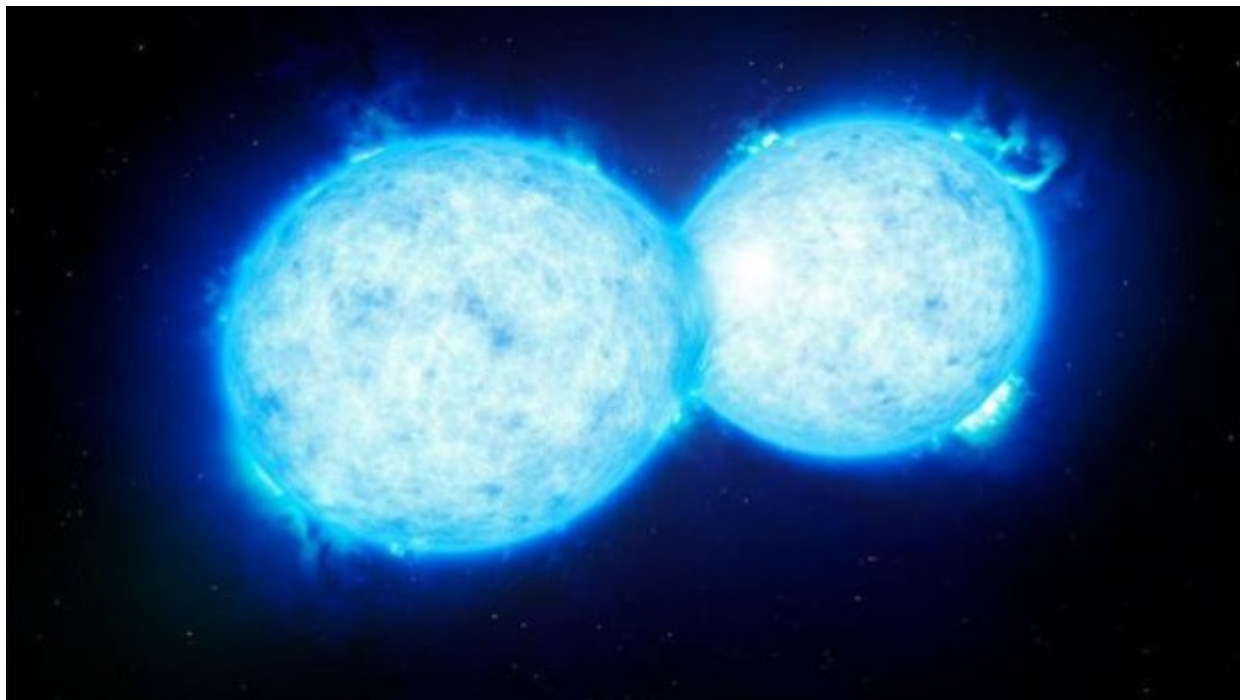
α δύο άστρα βρίσκονται ήδη τόσο κοντά ώστε οι ατμόσφαιρές τους πρέπει να έχουν συγχωνευτεί (Καλλιτεχνική απεικόνιση: ESO/L. Calçada)
